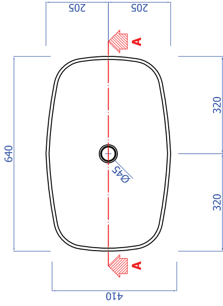
PIANTA
