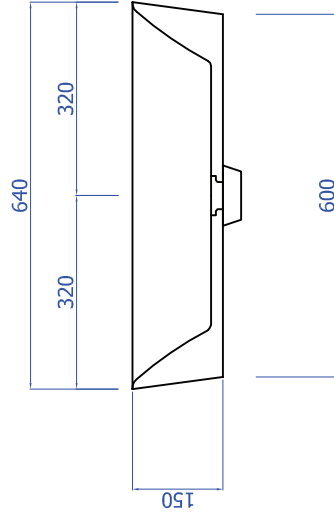
SEZIONE A-A
